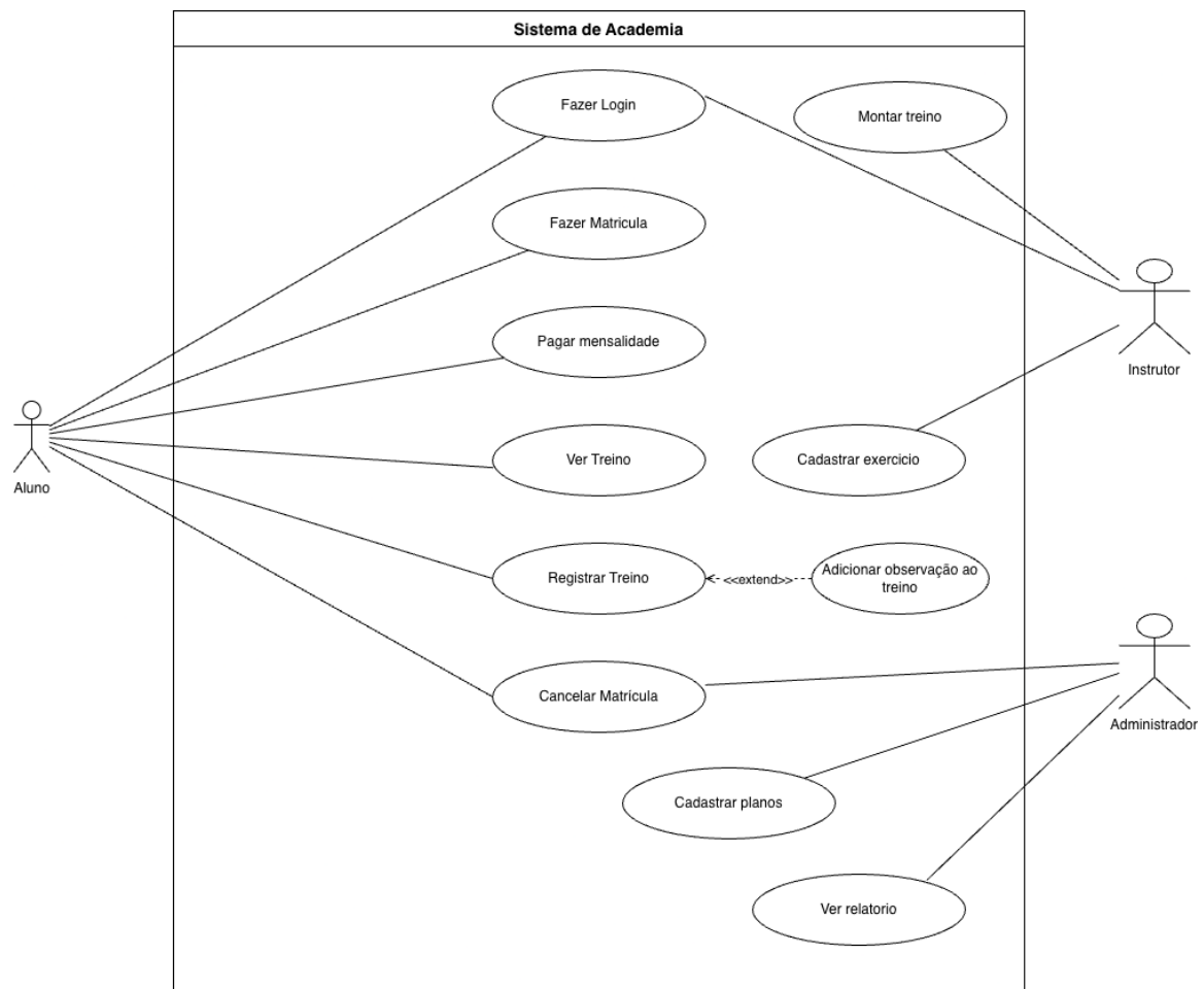
Figura 1: Diagrama de Caso de Uso – Sistema de Academia
