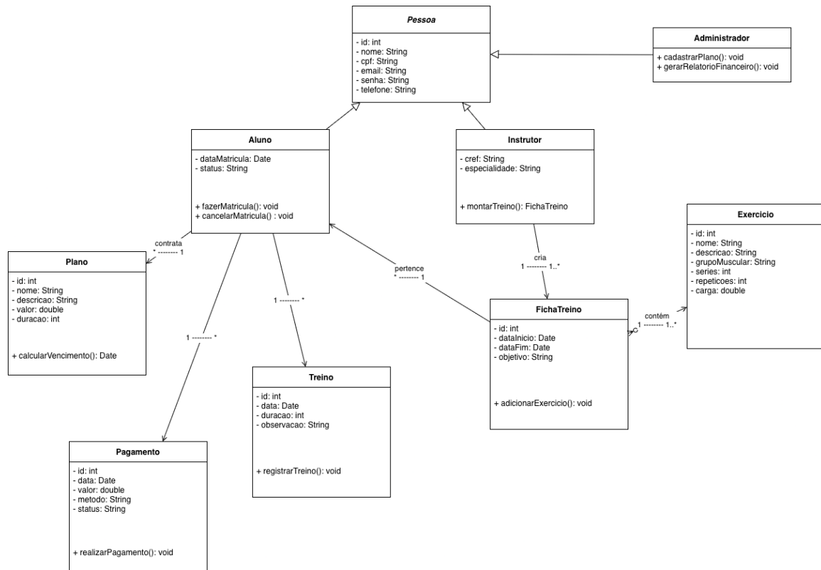
Figura 2: Diagrama de Classes – Sistema de Academia
