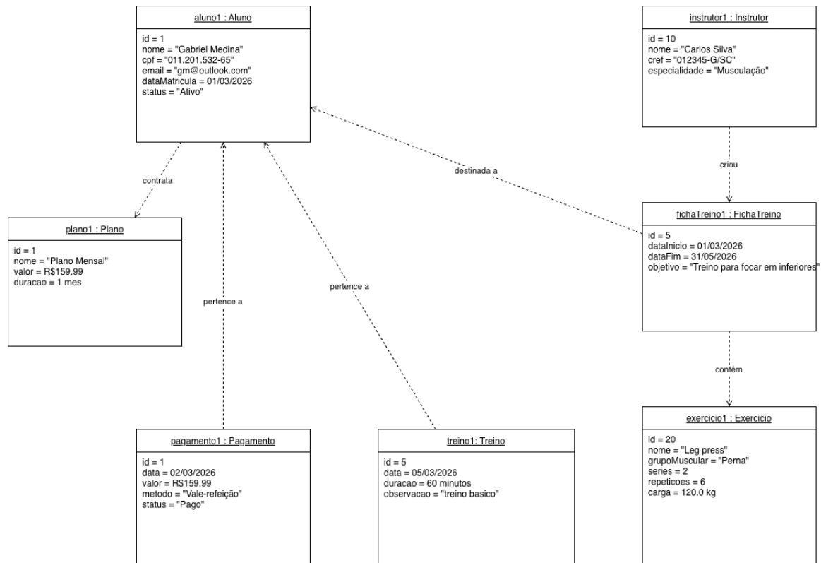
Figura 3: Diagrama de Objetos – Sistema de Academia
